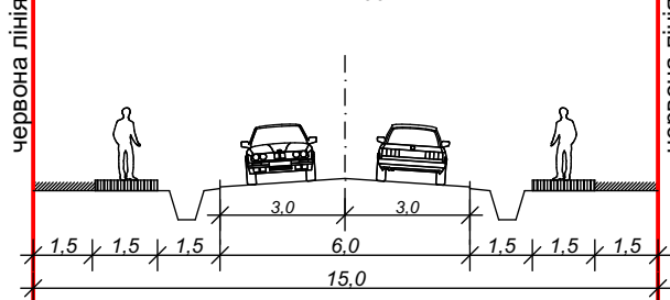
Поперечний профіль вул. Проектована 1, 3, 4, 5, 6 М 1:200
