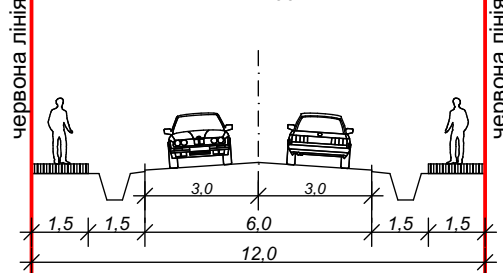
Поперечний профіль вул. Проектована 2 М 1:200
